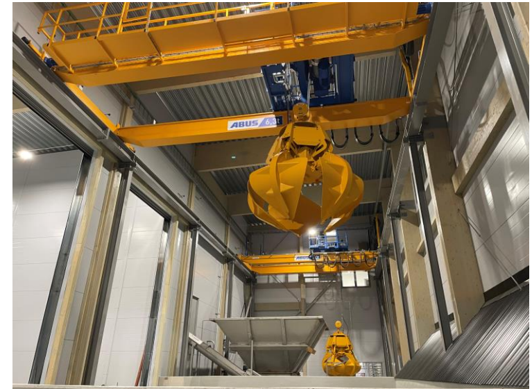
Travershall med gripklor monterade
